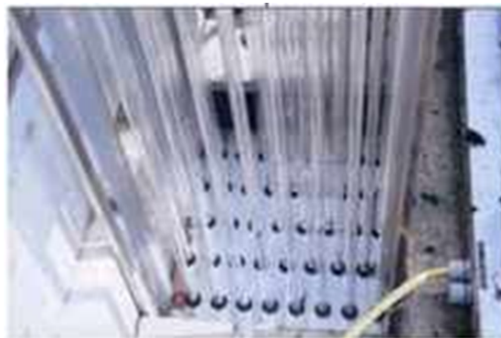
Figure 12 : Exemple de module de lampes verticales
