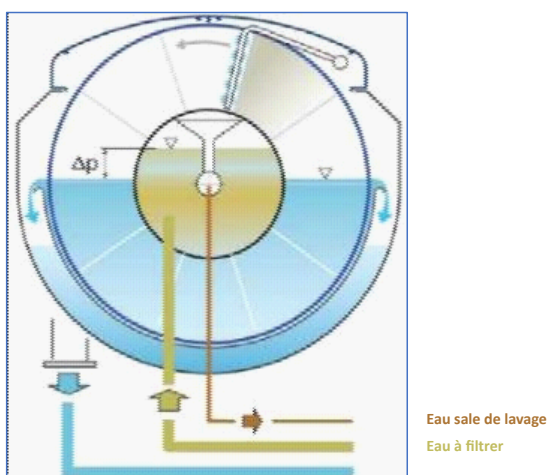
Figure 10 : Circuit des différentes eaux (propre et sale)
