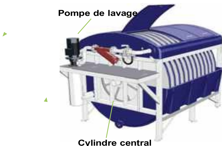
Figure 9 : Schéma d'un CompakblueTM avec un capot ouvert montrant le haut des disques
