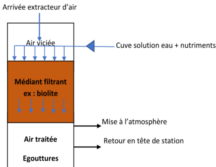
Figure 13 : Schéma de principe de traitement d'odeur
