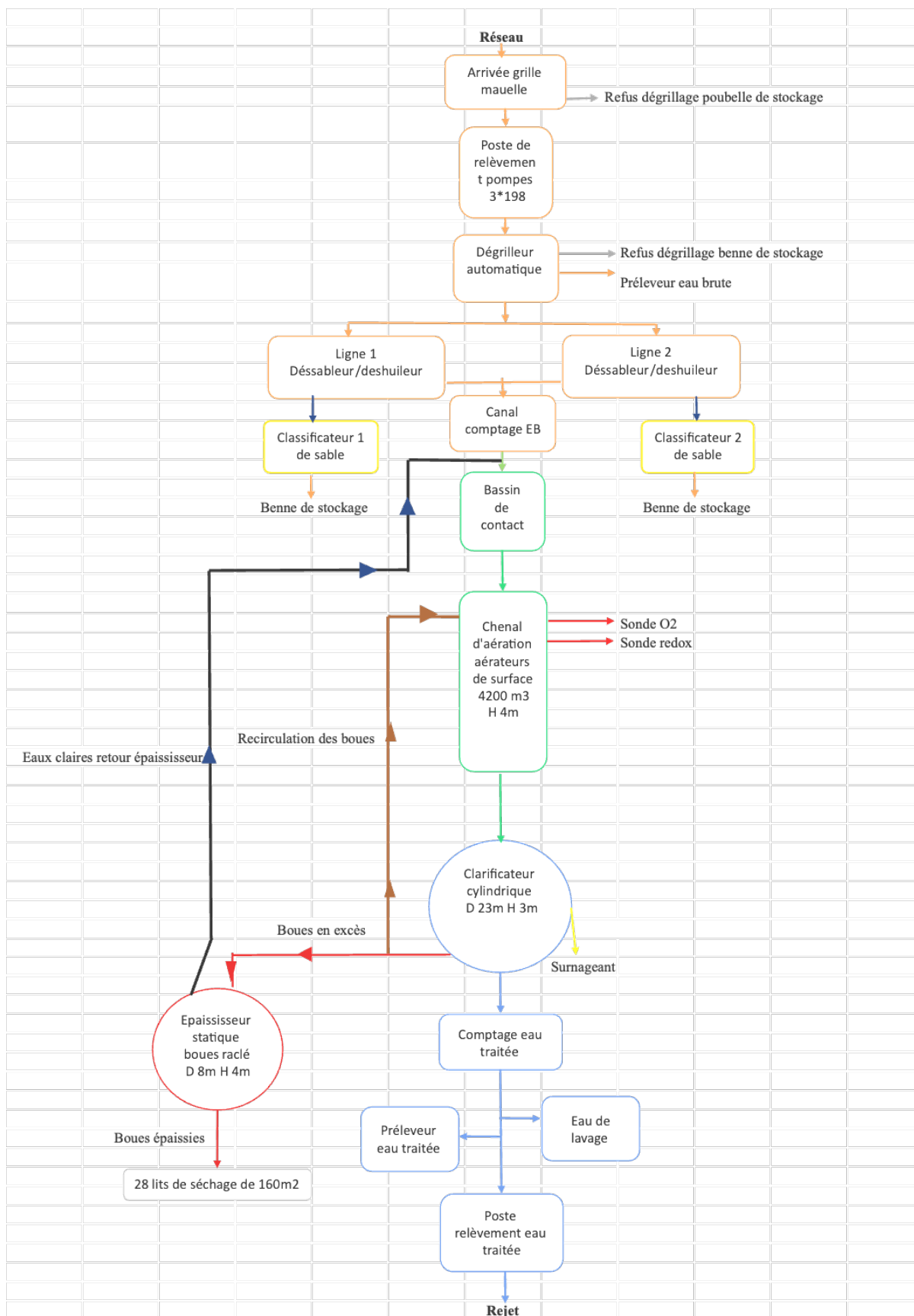
Figure 7 : Synoptique de fonctionnement de la STEP Mareth-Zarat
