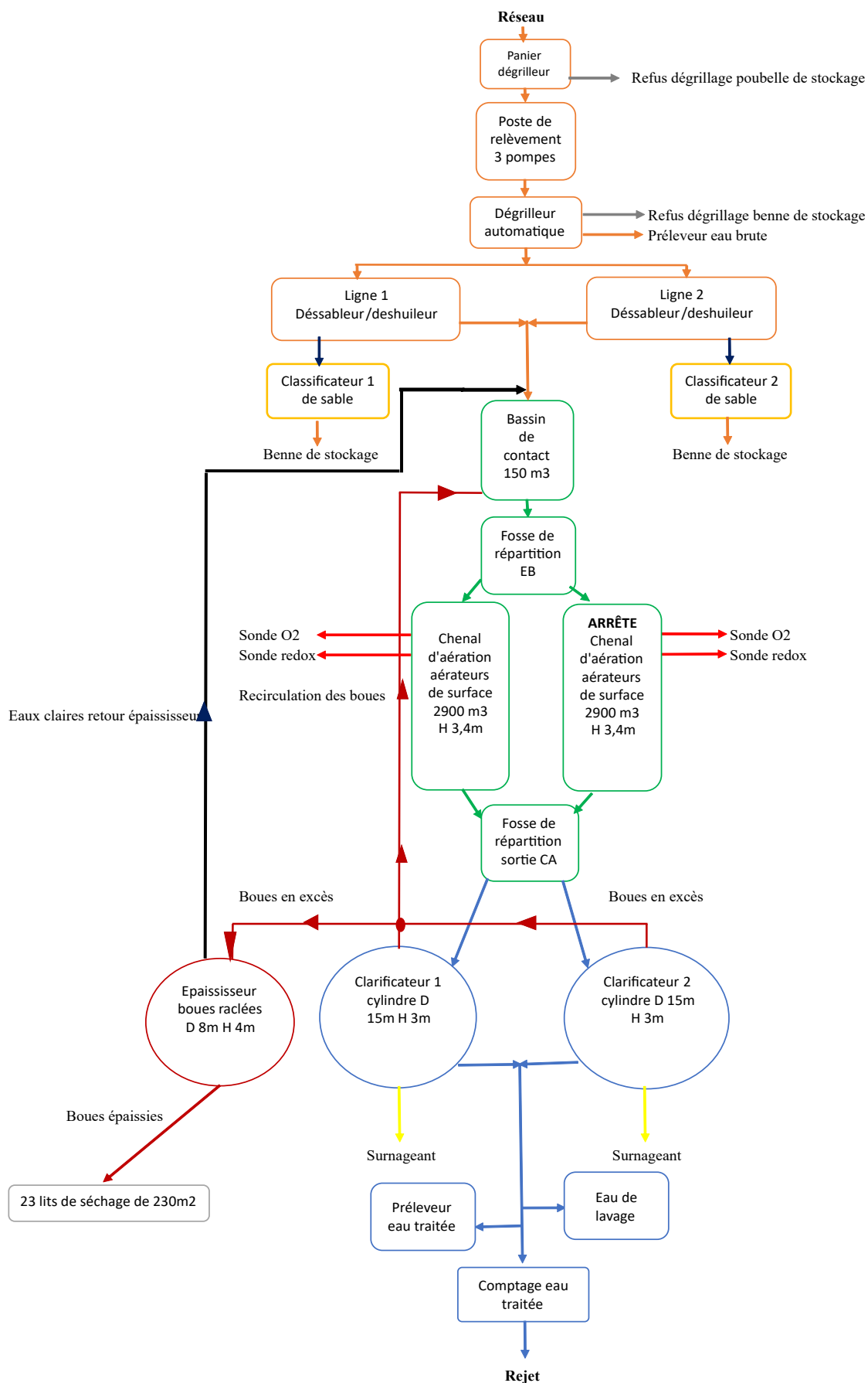
Figure 5 : Synoptique de fonctionnement de la STEP de Hamma
