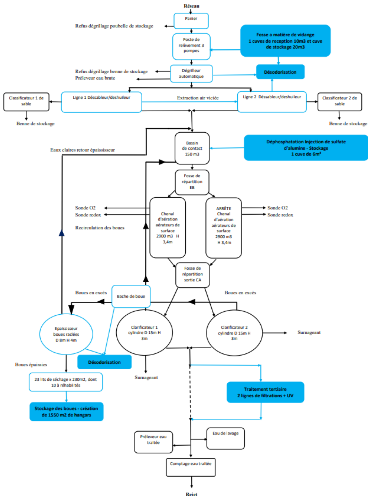
Figure 17 : Schéma global de fonctionnement la STEP de Hamma suite aux aménagements projetés
