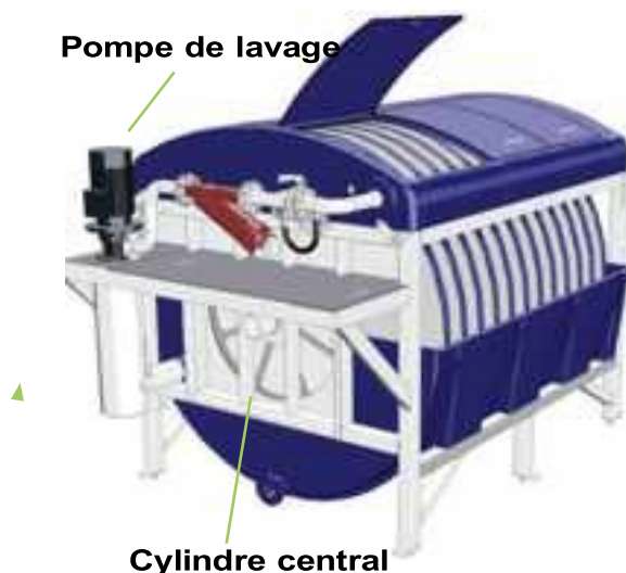
Figure 11 : Schéma d'un Compakblue™ avec un capot ouvert montrant le haut des disques
