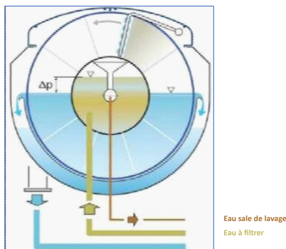
Figure 12 : Circuit des différentes eaux (propre et sale)
