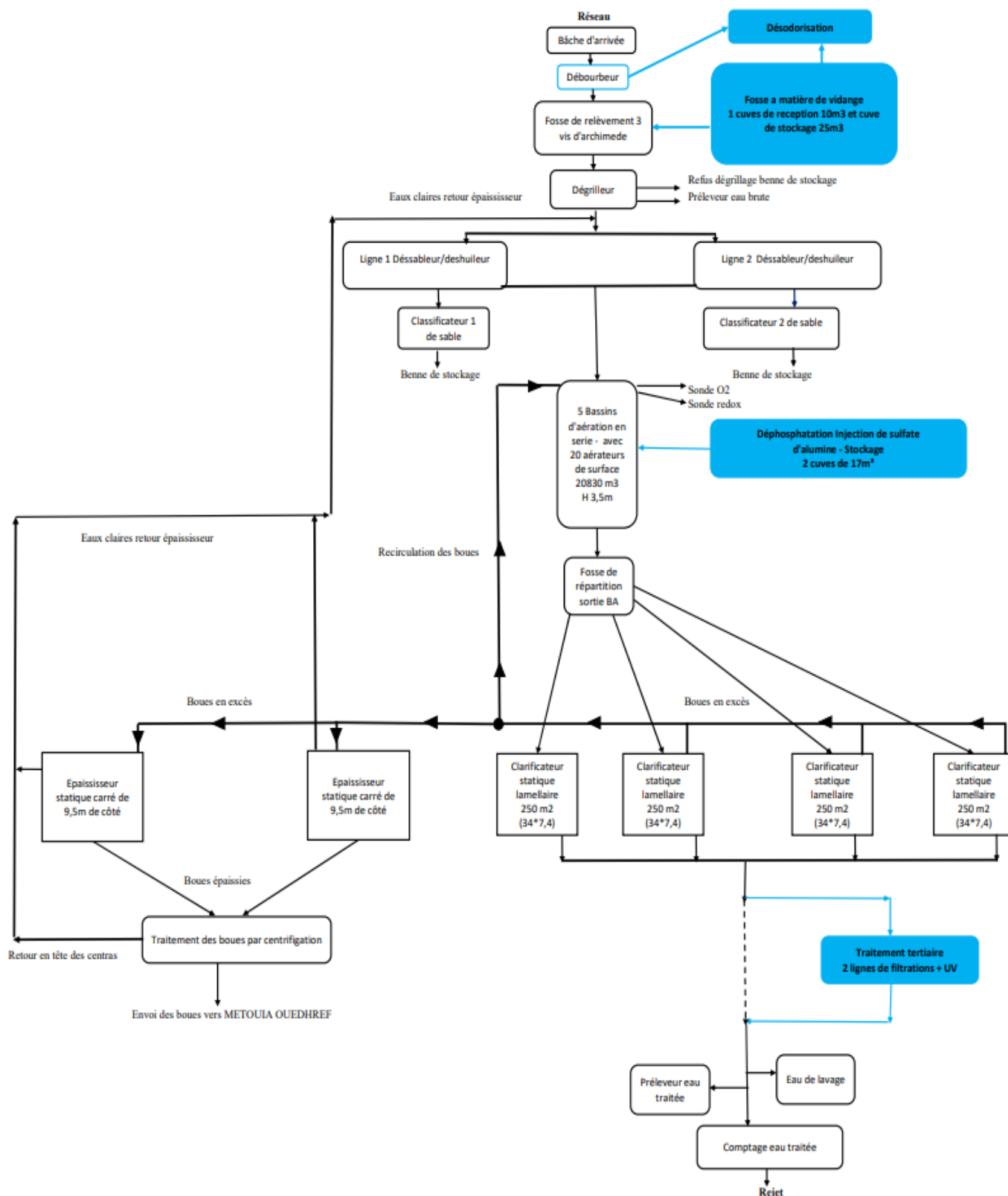
Figure 21 : Schéma global de fonctionnement la STEP de Gabès suite aux aménagements projetés
