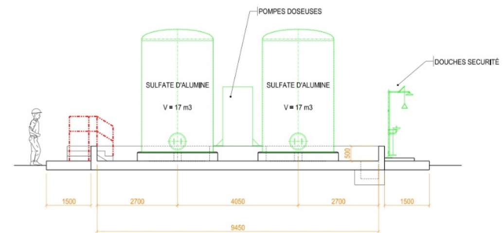
COUPE A-A
