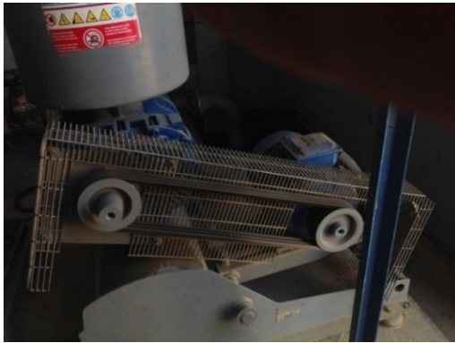
Surpresseur Hibon pour dégraisseur
