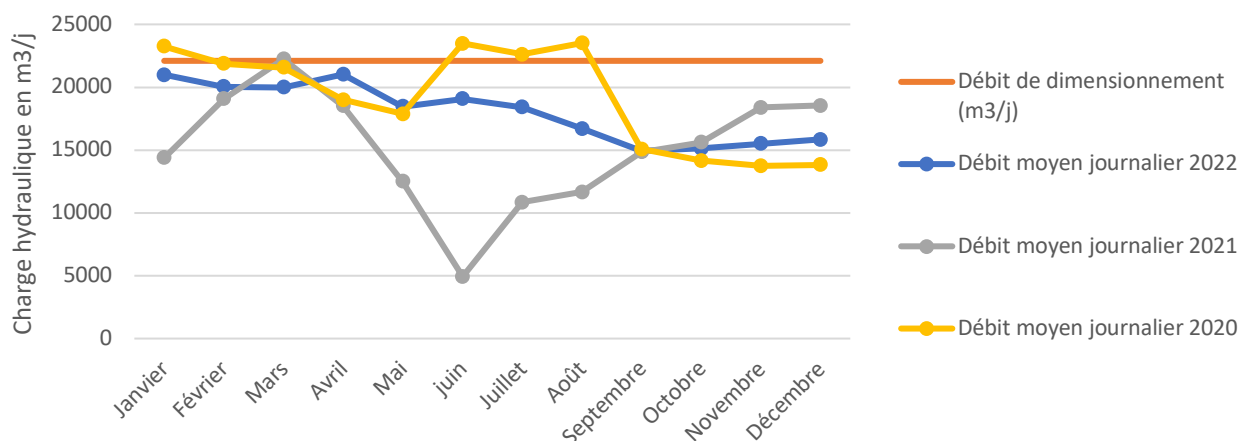
Figure 10 : Variation mensuelle du débit moyen journalier enregistré entre 2020 et 2022
