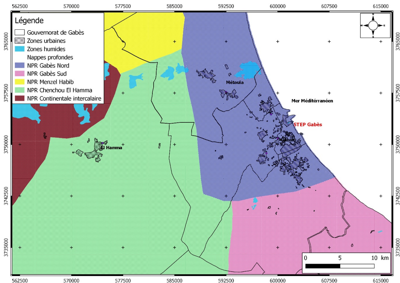
Figure 29 : Nappes profondes de la zone d'étude (carte agricole de Gabès, 2002)
