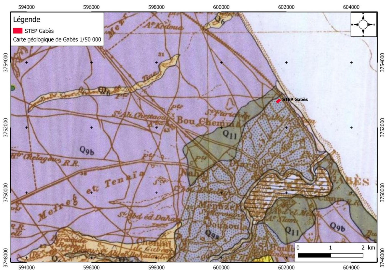
Figure 25: Extrait de la carte géologique de Gabès au 1/50 000
