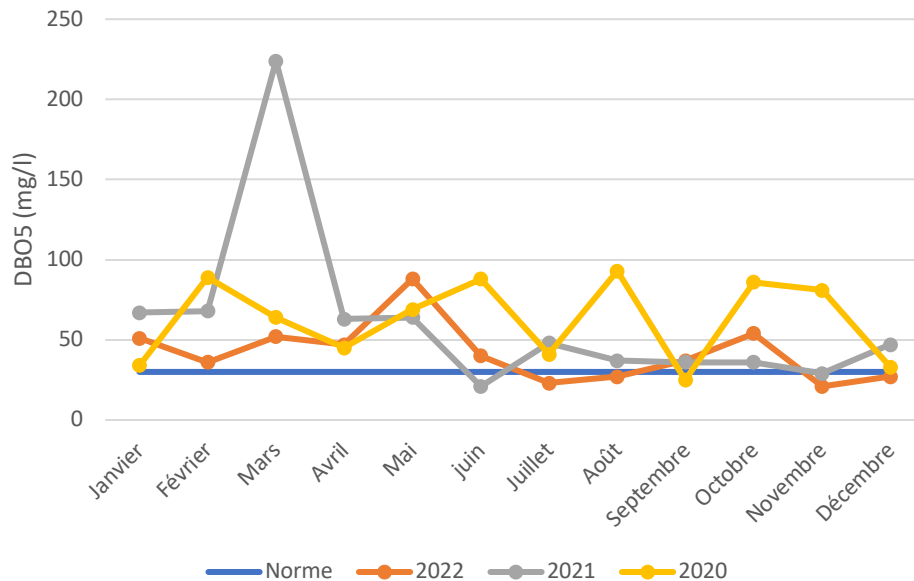
Figure 12 : Variation mensuelle des concentrations moyennes des eaux usées traitées en DBO5
