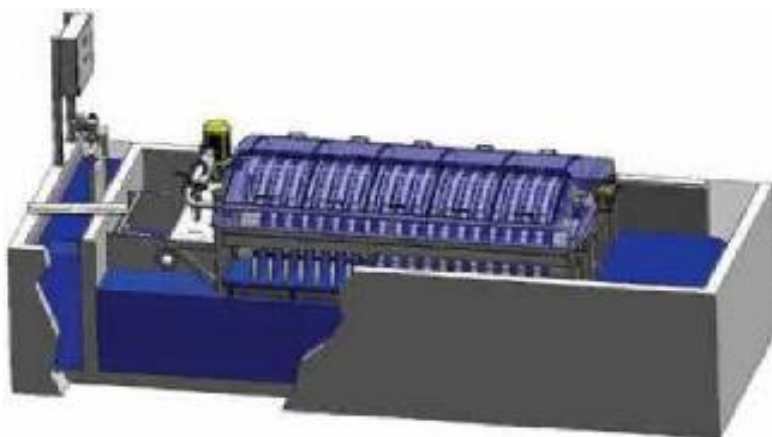
Figure 15 - Exemple d'appareil à installer en cuve béton
