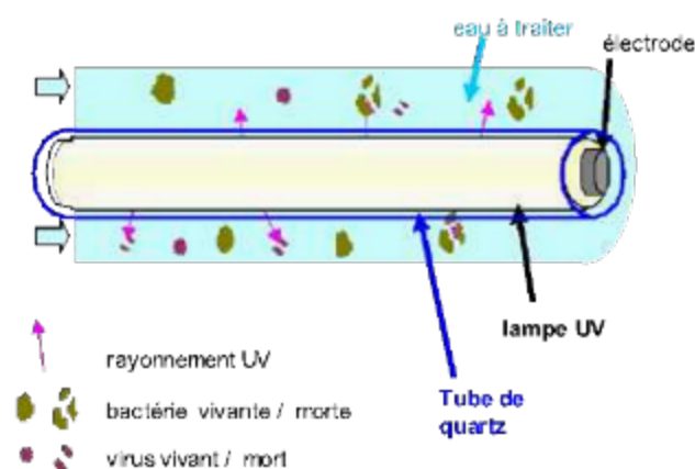
Figure 18 : Schéma de fonctionnement des lampes UV
