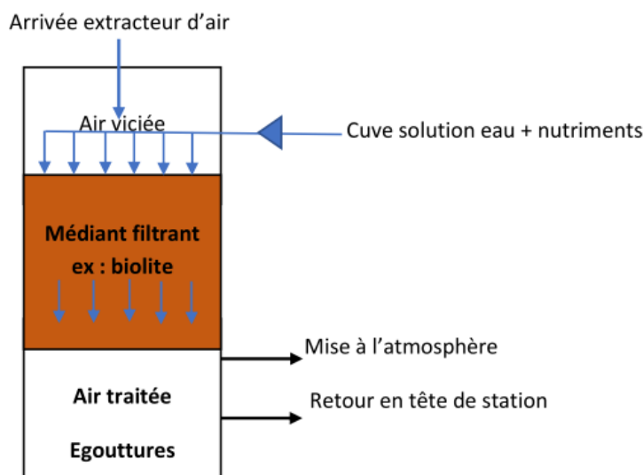
Figure 20 : Schéma de principe de traitement d'odeur
