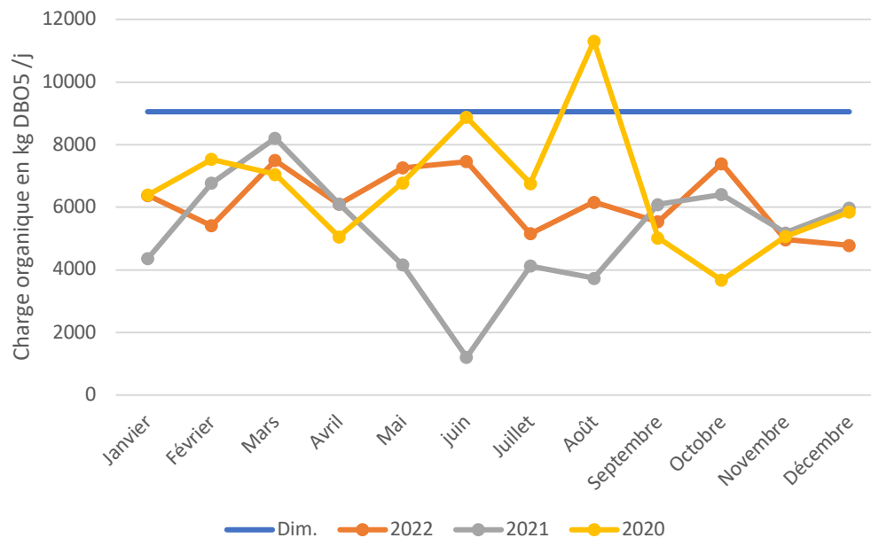
Figure 11 : Variation mensuelle de la charge journalière moyenne enregistrée entre 2020 et 2022
