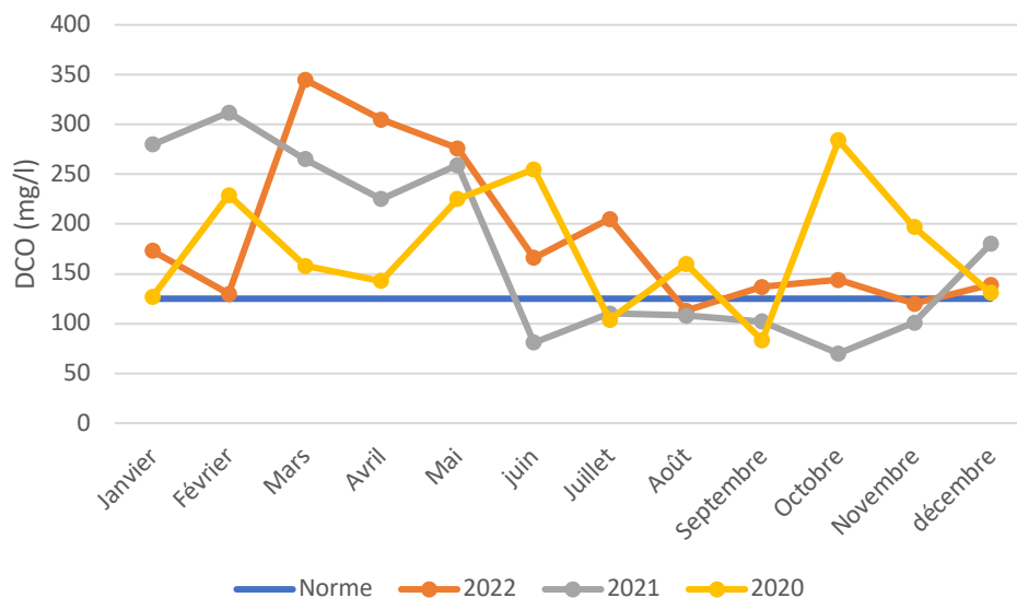
Figure 13 : Variation mensuelle des concentrations moyennes des eaux usées traitées en DCO
