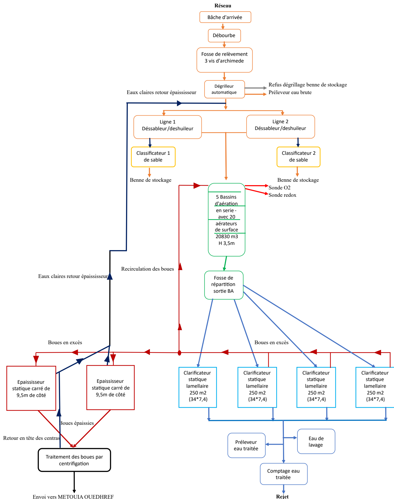
Figure 9 : Synoptique de fonctionnement de la STEP de Gabès
