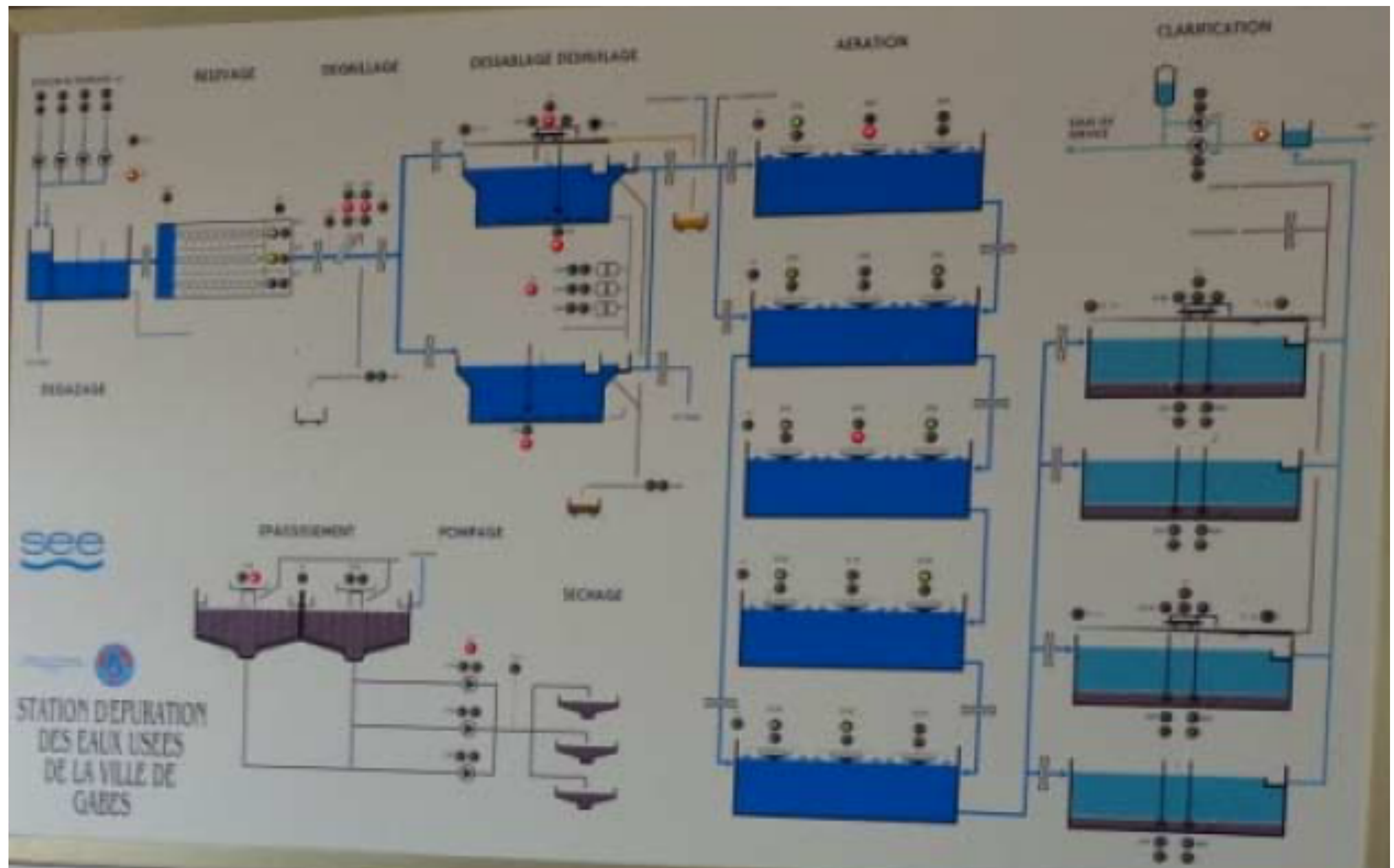
Figure 8 : Schéma d'ensemble de la STEP de Gabès
