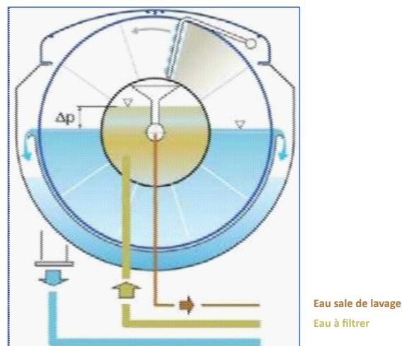
Figure 17 - Circuit des différentes eaux (propre et sale)
