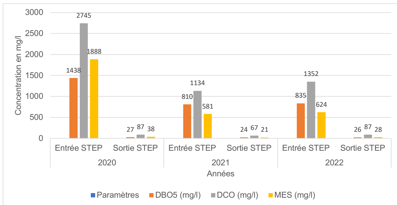
Figure 24 : Concentrations annuelles moyennes : DBO 5 , DCO et MES (SEGOR : Rapports mensuels d'exploitation de la STEP El Hancha)
