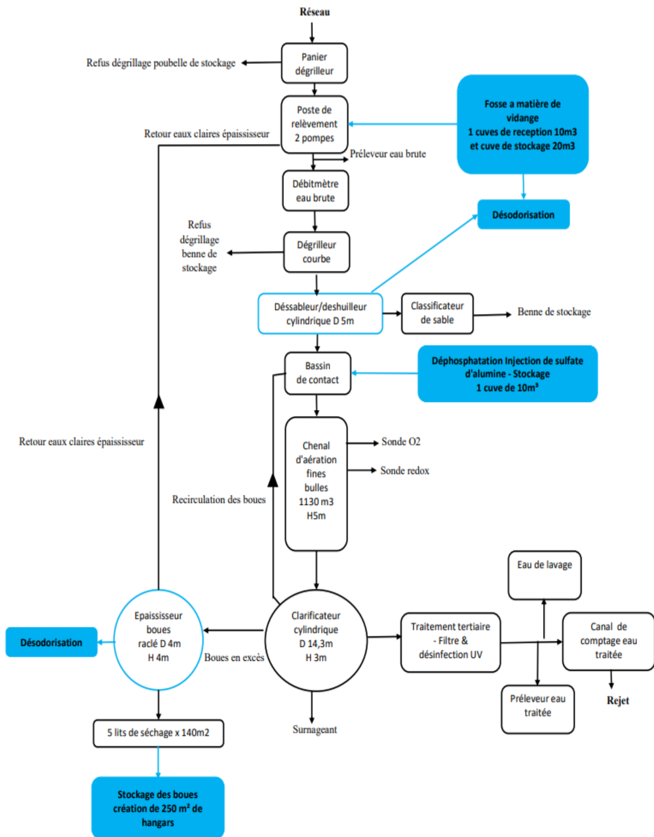
Figure 28 : Schéma global de fonctionnement la STEP El Hancha suite aux aménagements projetés
