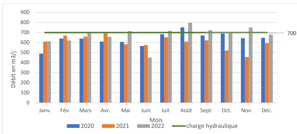
Figure 23 : Charges hydrauliques de la STEP d'El Hancha (SEGOR : Rapports mensuels d'exploitation d'El Hancha)
