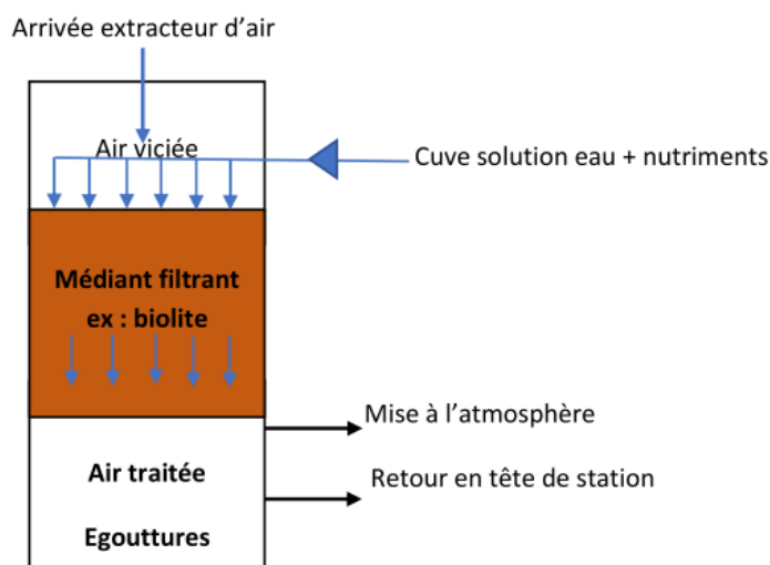
Figure 26 : Schéma de principe de traitement d'odeur
