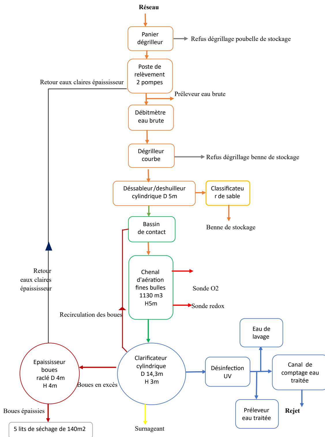
Figure 8 : Synoptique de fonctionnement de la STEP d'El Hancha
