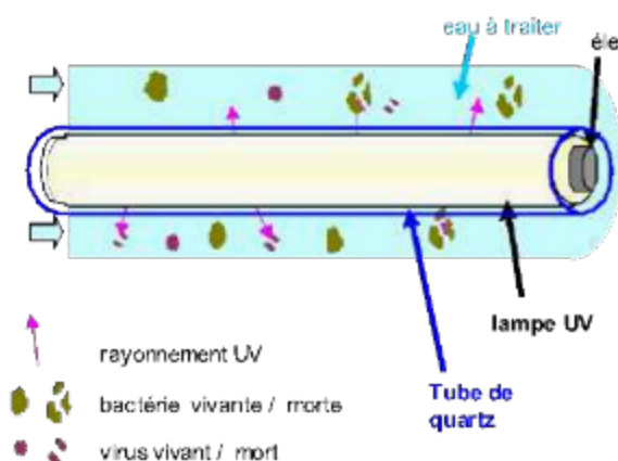
Figure 15 : Schéma de fonctionnement des lampes UV
