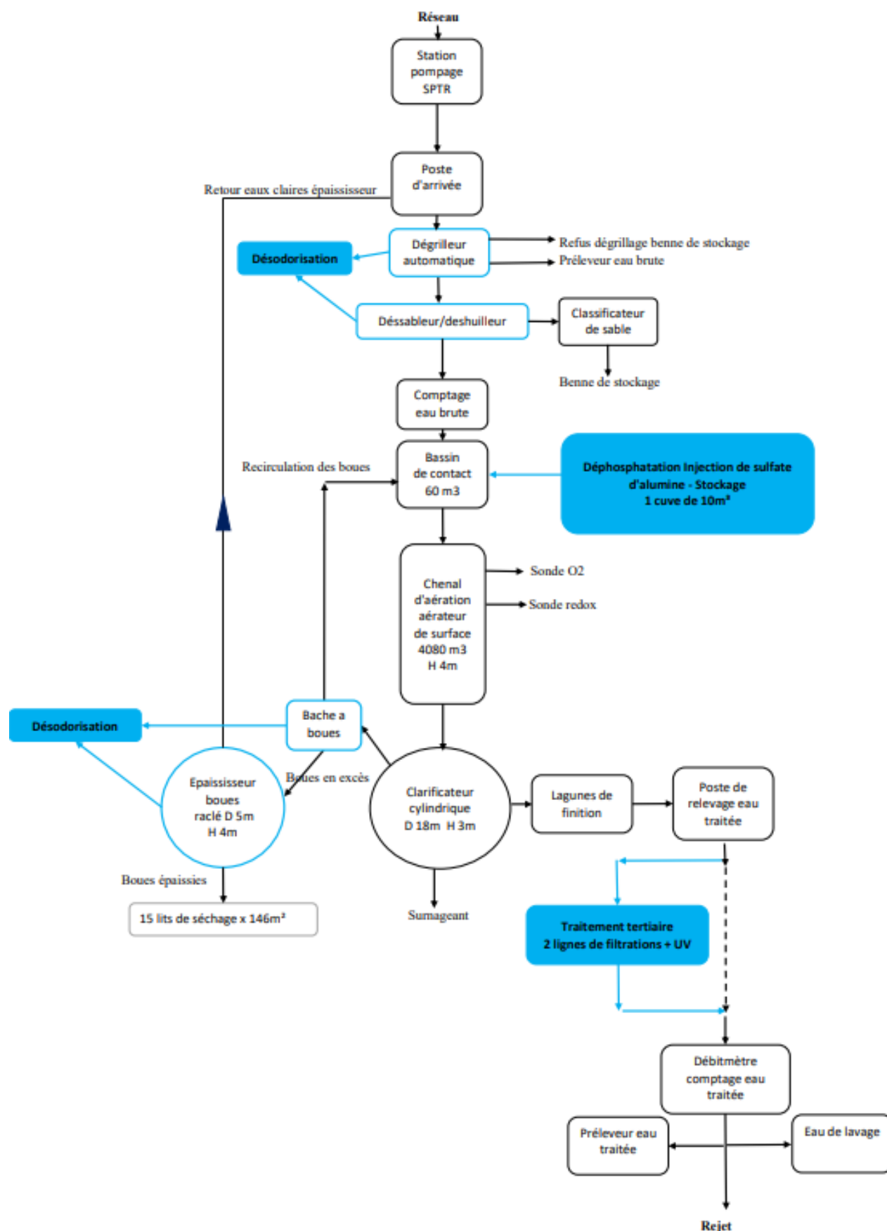
Figure 18 : Synoptique de fonctionnement de la STEP après travaux
