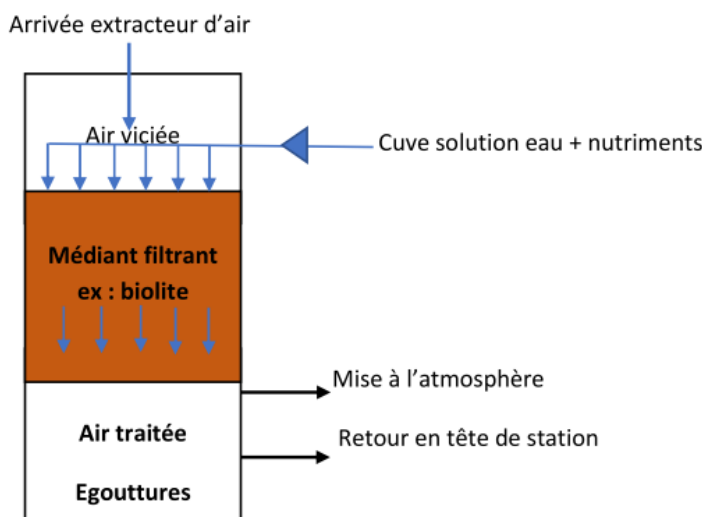
Figure 17 : Schéma de principe de traitement d'odeur
