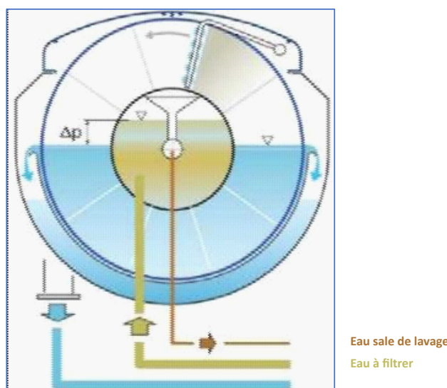
Figure 14 - Circuit des différentes eaux (propre et sale)
