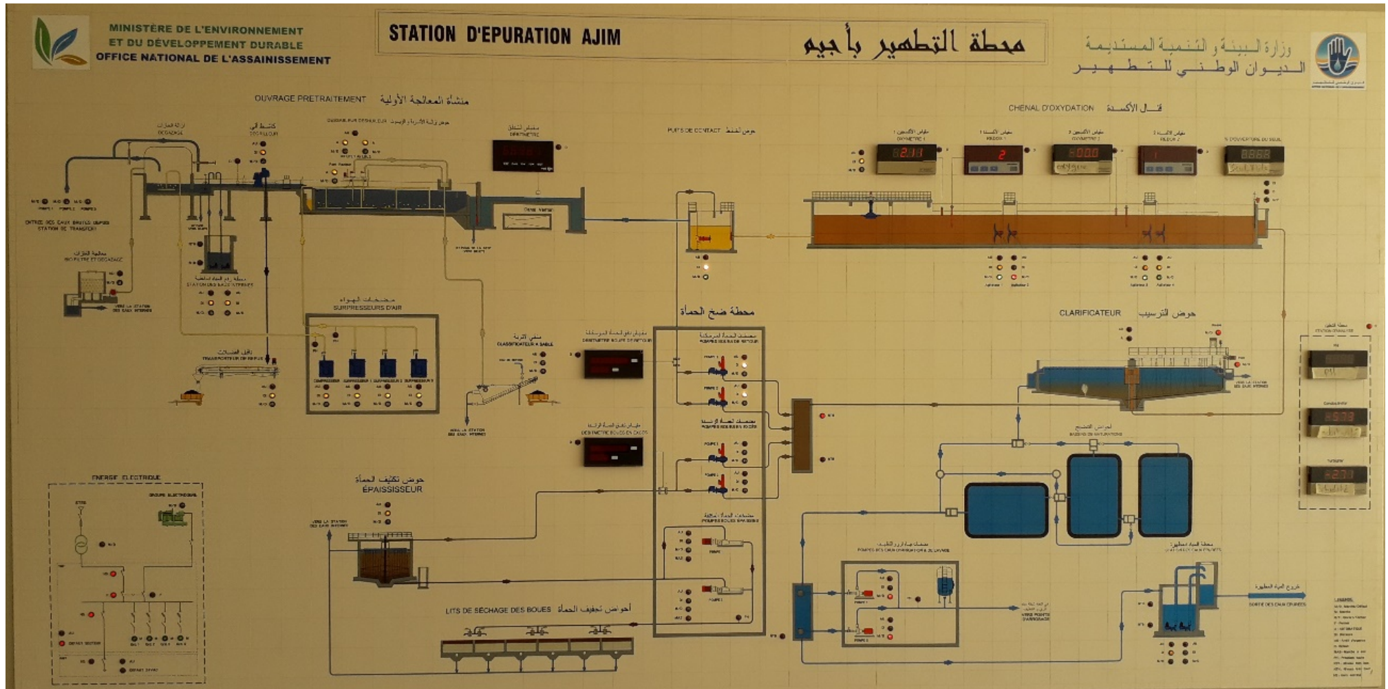
Figure 10 : Schéma d'ensemble de la STEP de Djerba-Ajim
