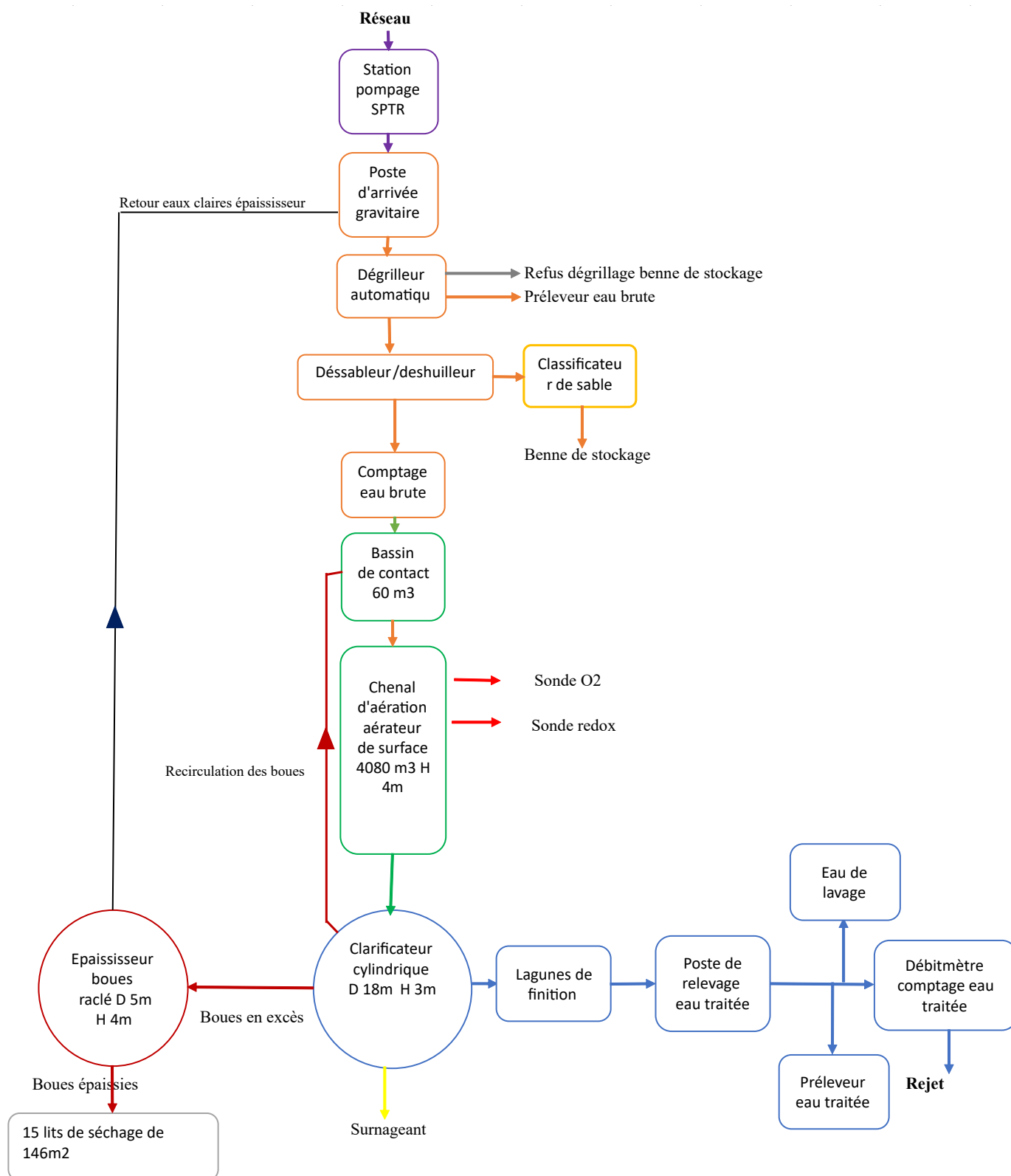
Figure 11 : Synoptique de fonctionnement de la STEP Djerba-Ajim
