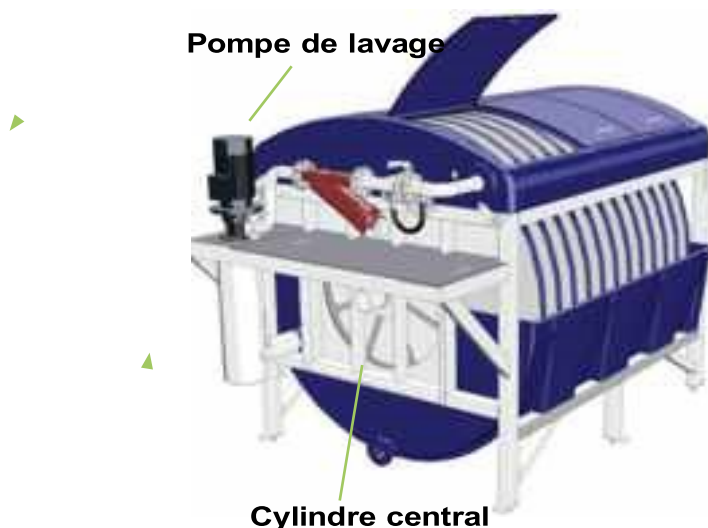
Figure 13 Schéma d'un CompakblueTM avec un capot ouvert montrant le haut des disques
