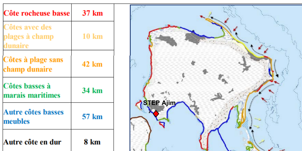
Figure 22 : Les différents faciès morphologiques de l'île de Djerba (IHE, 2015)
